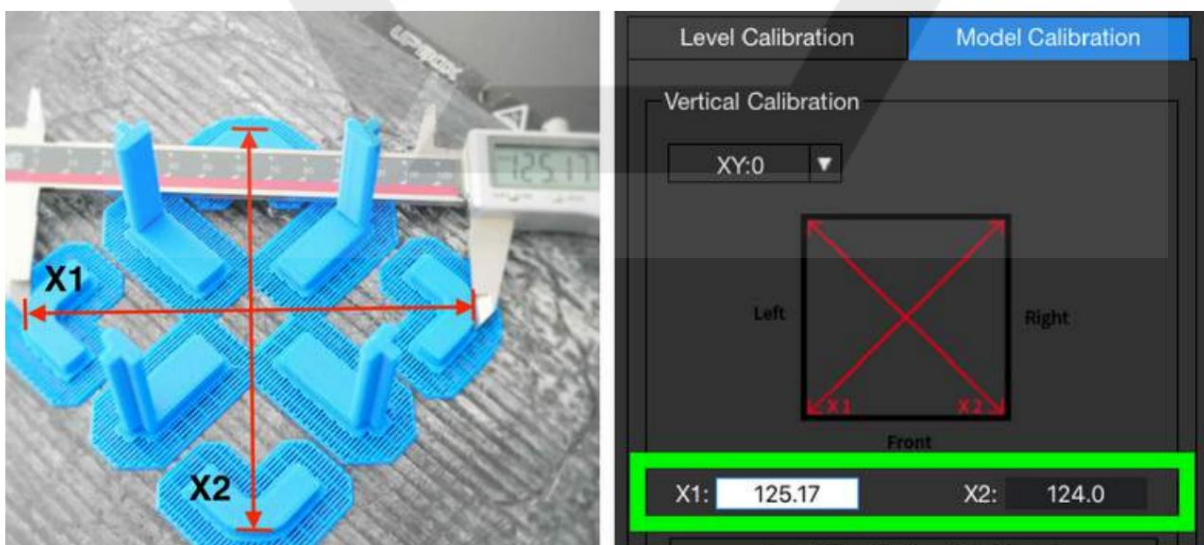
Figure 6.23 Étalonnage de l'axe X/Y
