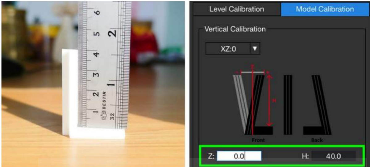
Figure 6.24 Étalonnage de l'axe X/Y
