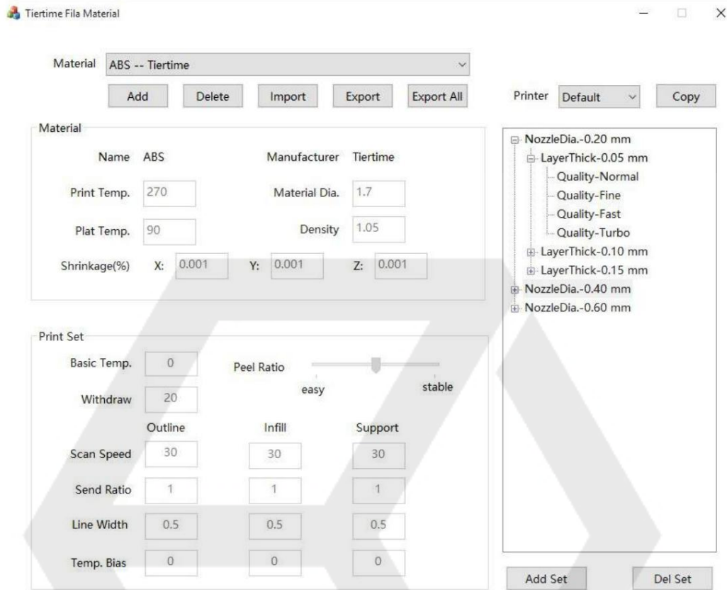
Figure 6.16 Profil de filament personnalisé
